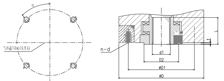
推力型连接尺寸图 Thrust type connection size chart
