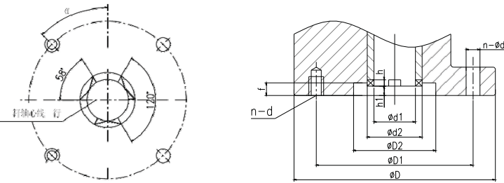
转矩型连接尺寸图 Torque type connection size chart
