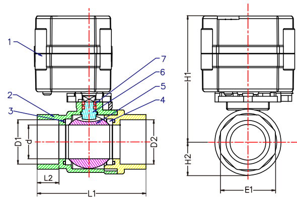
外形尺寸图 Outline Size Dimension
