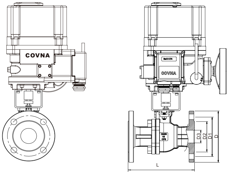
主要外形及连接法兰尺寸 ANSI-150# Main Outline and Connecting Flange Size
