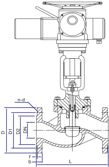
电动截止阀主要外形及连接尺寸(国标) Main Outline and Connecting ( GB )
