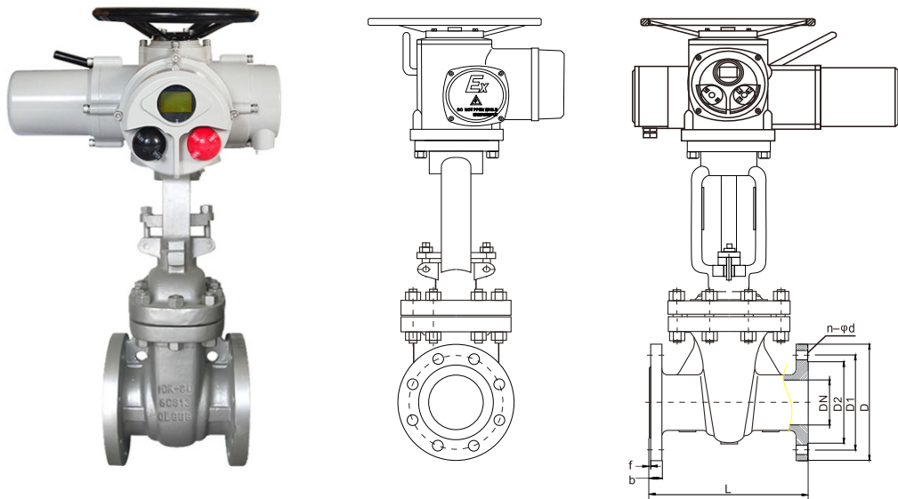
电动闸阀主要外形及连接尺寸(日标) Main Outline and Connecting（JIS）
