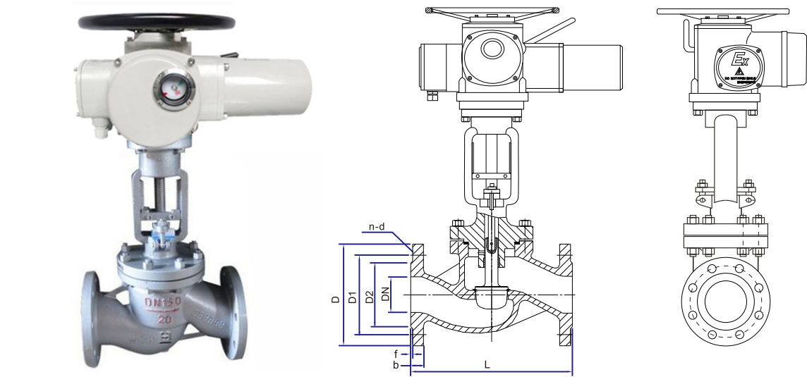
电动闸阀主要外形及连接尺寸(日标) Main Outline and Connecting（JIS）
