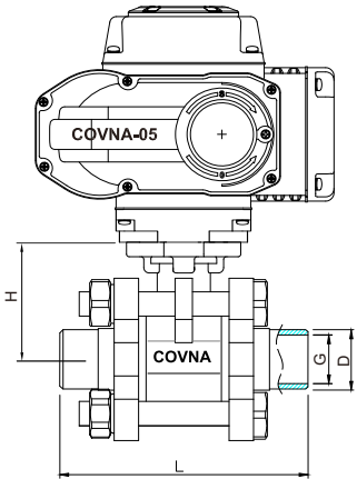
焊接型 Welded Type
